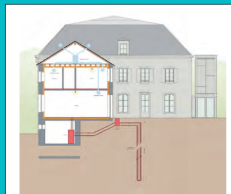
coupes techniques
