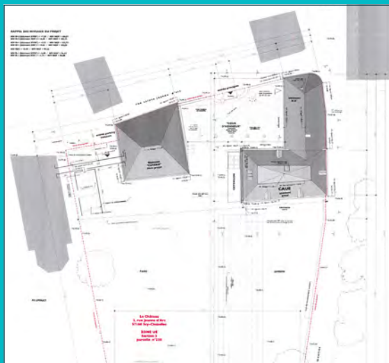
plan masse
